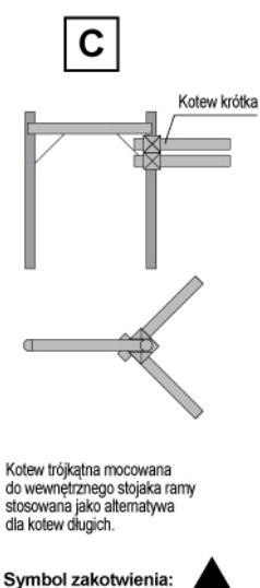
Rys. 10. Rodzaje kotew
